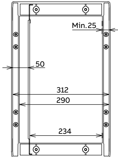
Beschikbare ruimte bij gebruik van binnendeur
