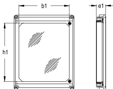
Klapdeksel transparant
