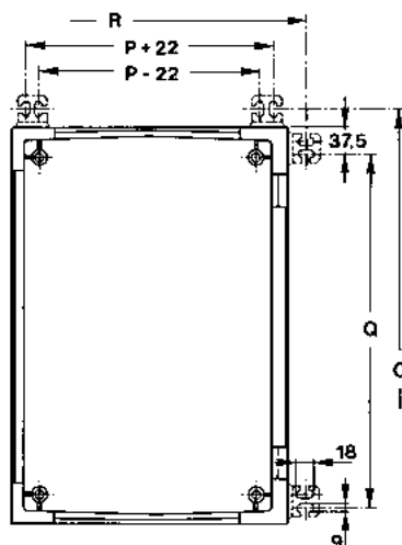
Met roestvaststalen bevestigingsvoetjes
