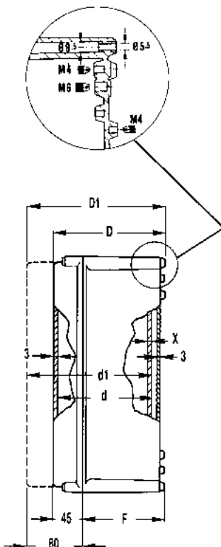
APO 11 Klapdeksel met flens
