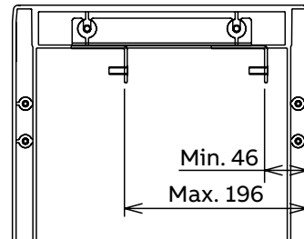
Verstelbare montageplaat
