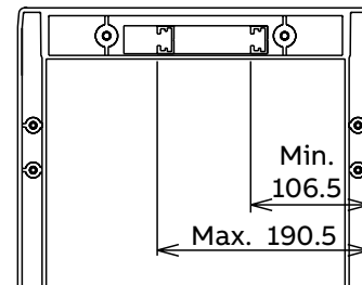
Montageframe traploos verstelbaar
