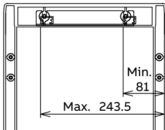
Montageframe in diepte van 12.5 mm verstelbaar
