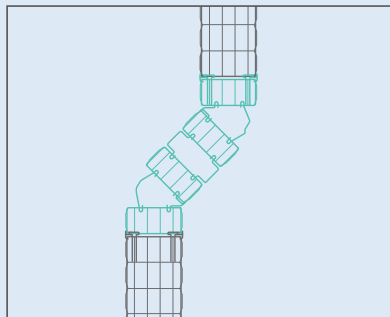
Voorbeeld van een configuratie met 1 Cablobend
